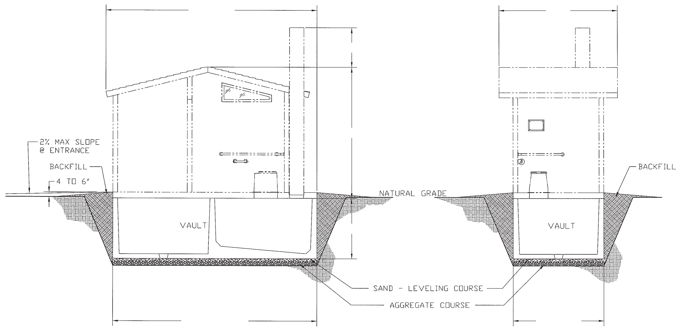
SIDE EVLEVATION
